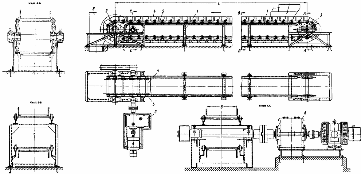
Şekil 6.1 Paletli konveyörler
