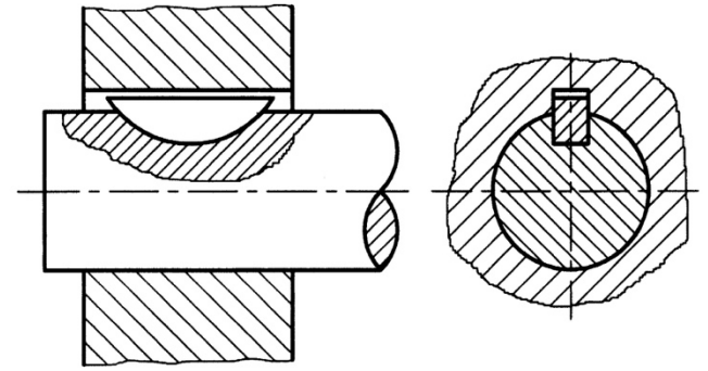
Yarım ay kama
