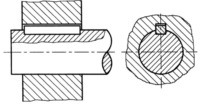
Eđimsiz (paralel yzeyli) boyuna kama
