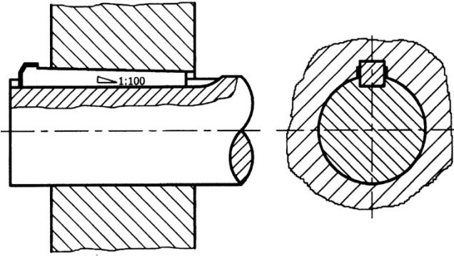
Eđimli Boyuna Burunlu Kama
