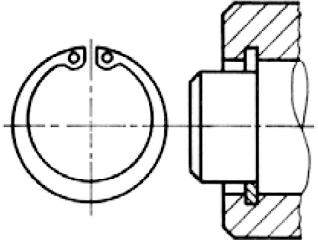
İç segman
