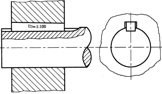
Eđimli Boyuna Burunlu Kama
